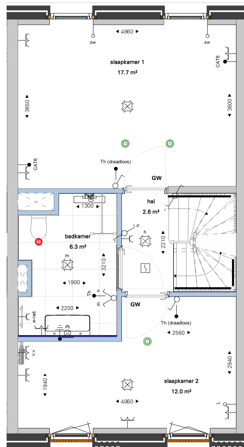
tweede verdieping
