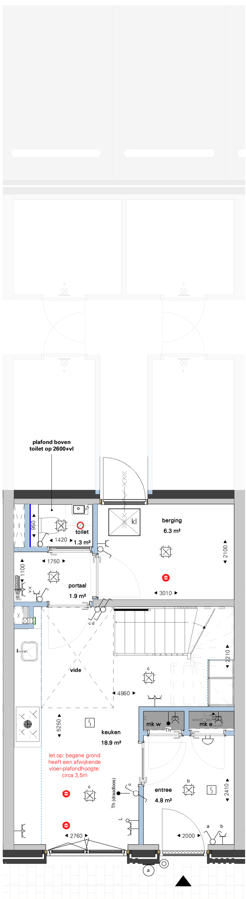
begane grond
