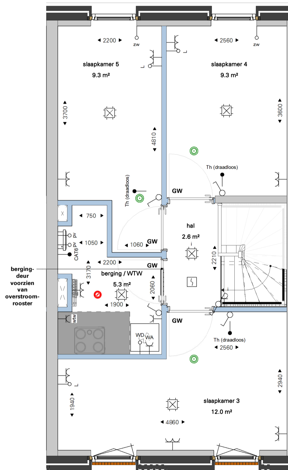
derde verdieping
