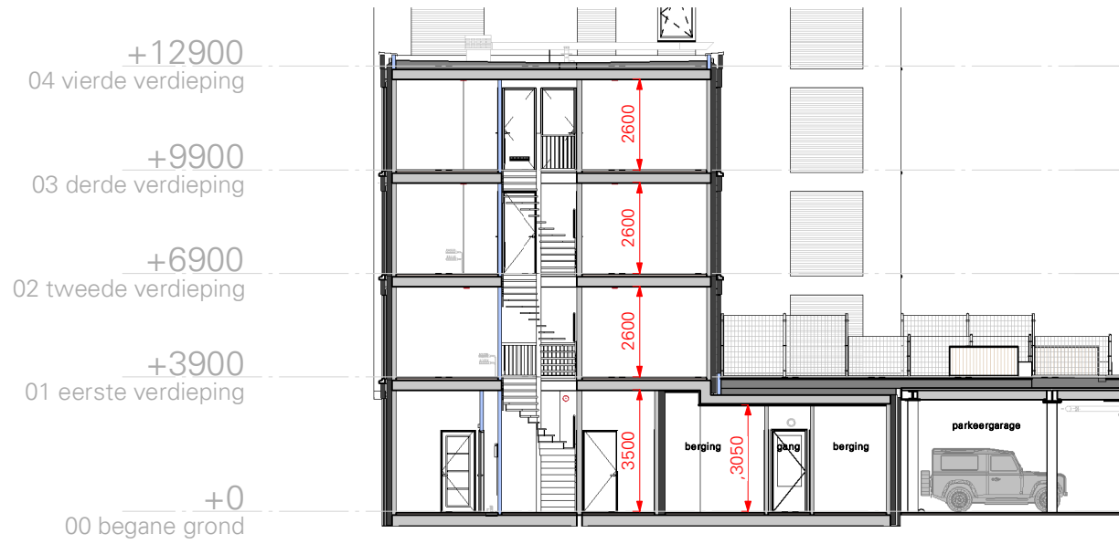
VK Doorsnede B3.A
