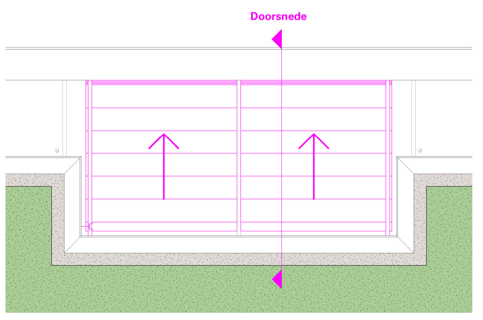
01.09.00.021 Bedienbaar harmonica schaduwdoek
