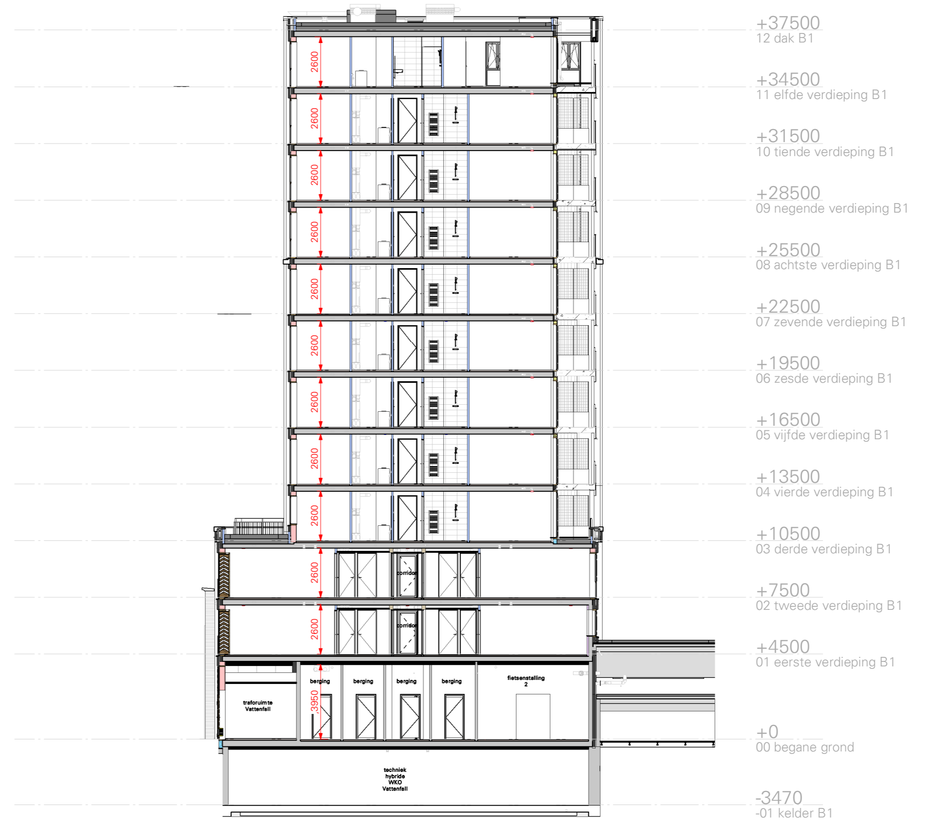
VK Doorsnede B1.D
