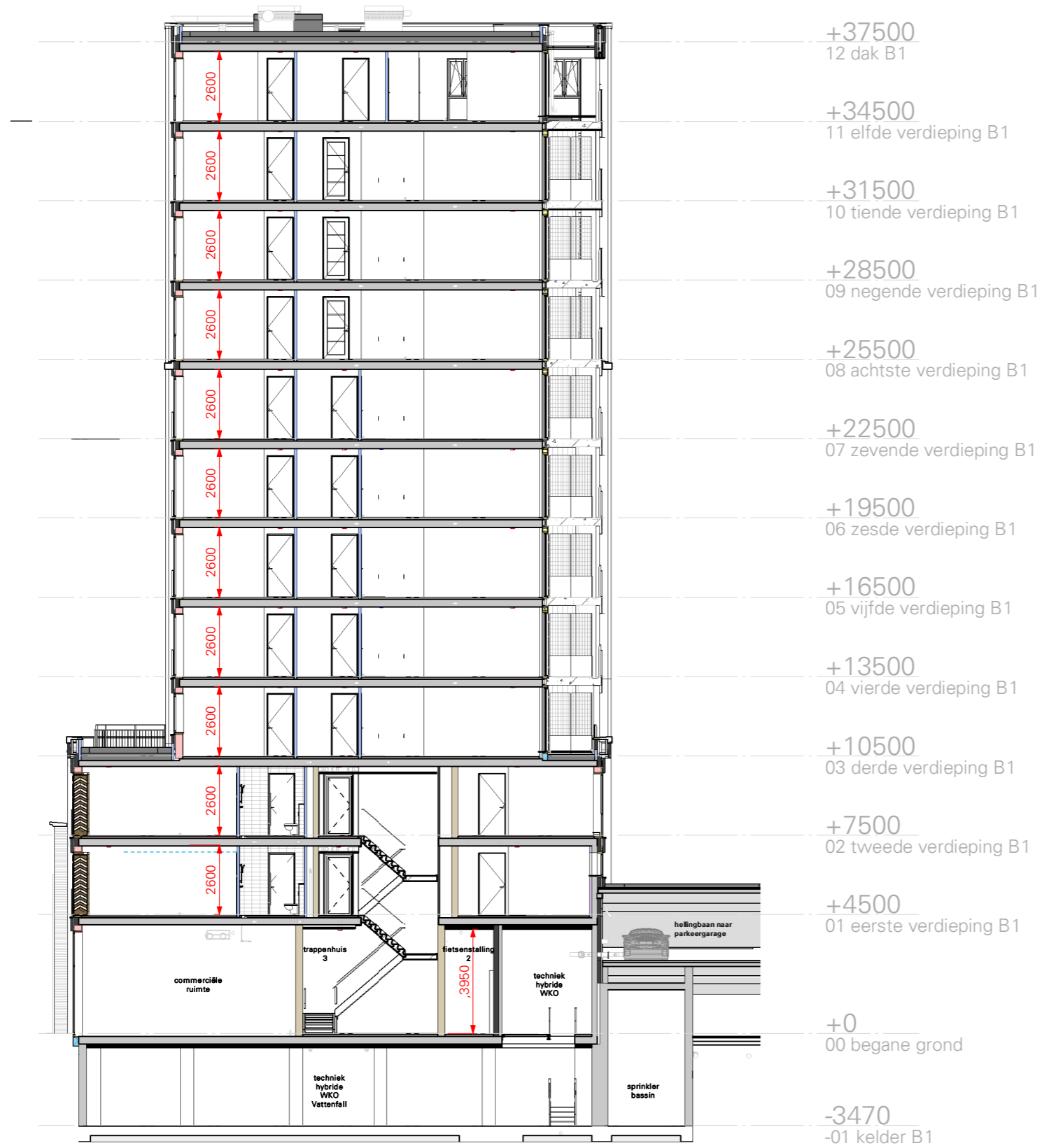
VK Doorsnede B1.C
