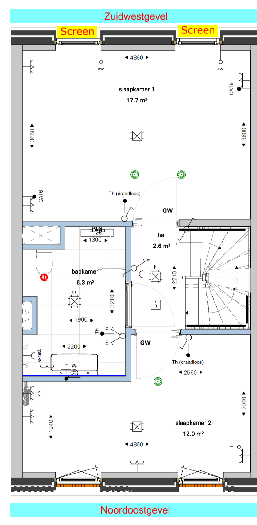
tweede verdieping
