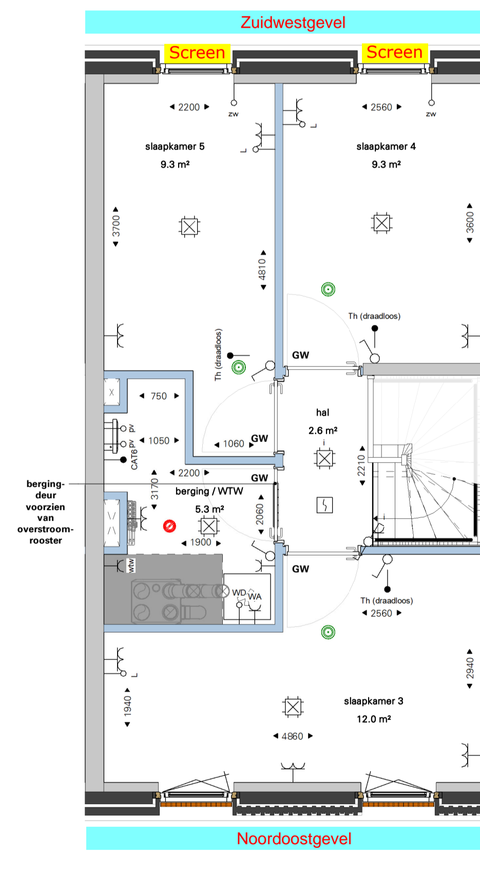
derde verdieping
